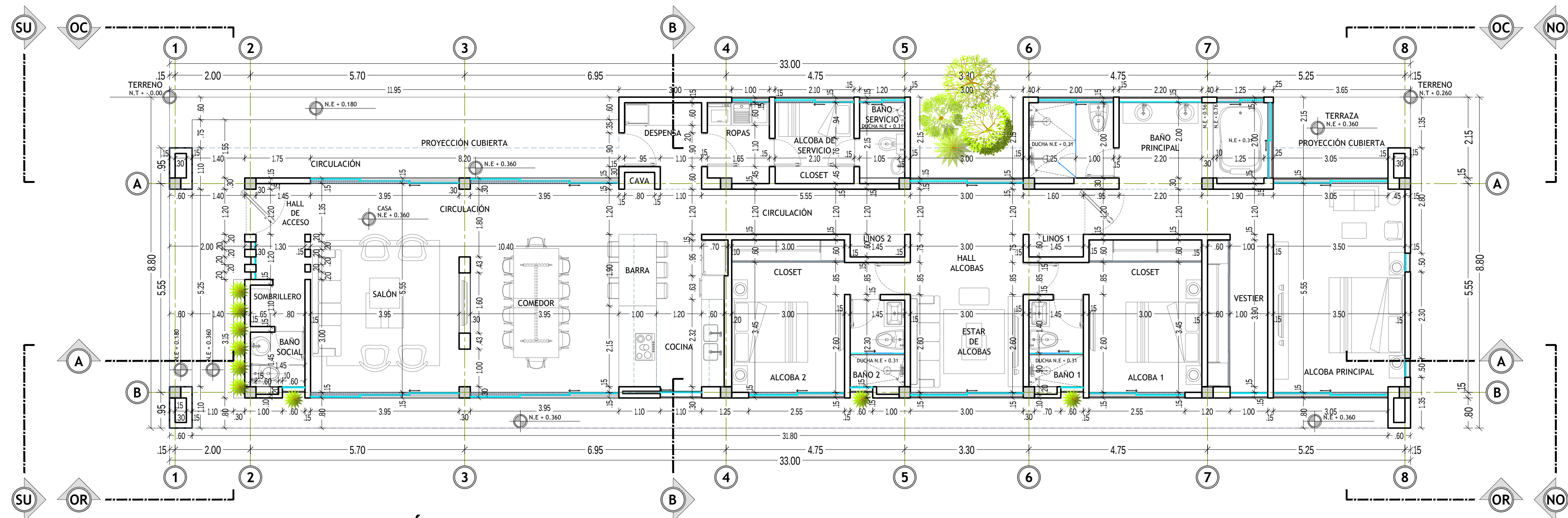
PLANTA ARQUITECTÓNICA - CASA
