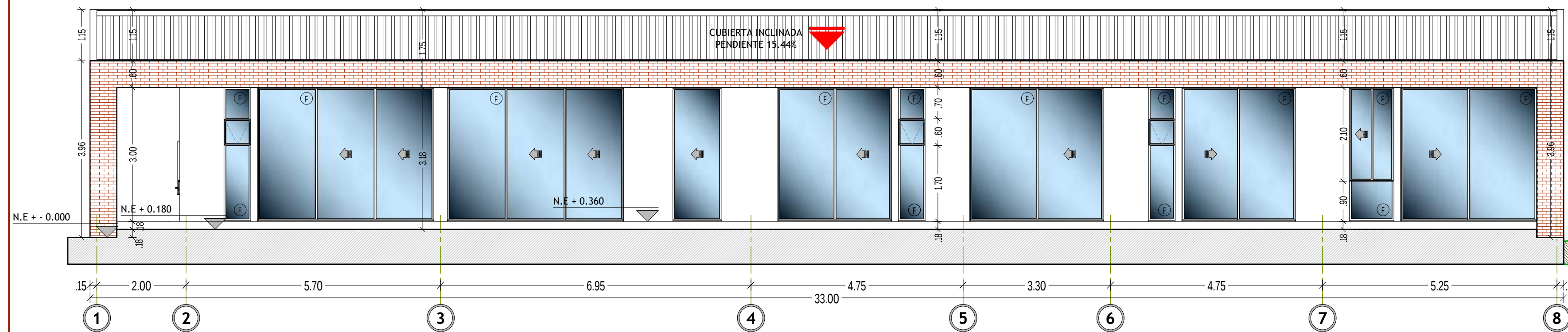
FACHADA SURORIENTE - OR
