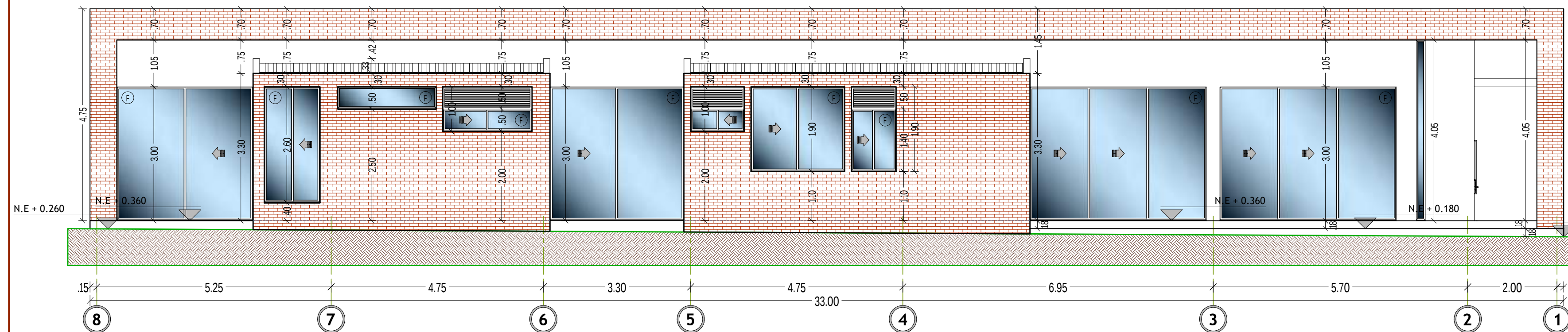
FACHADA NOROCCIDENTE - OC
