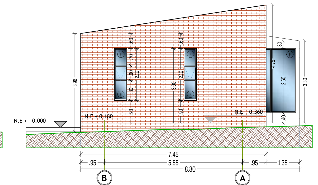
FACHADA NORORIENTE - NO
