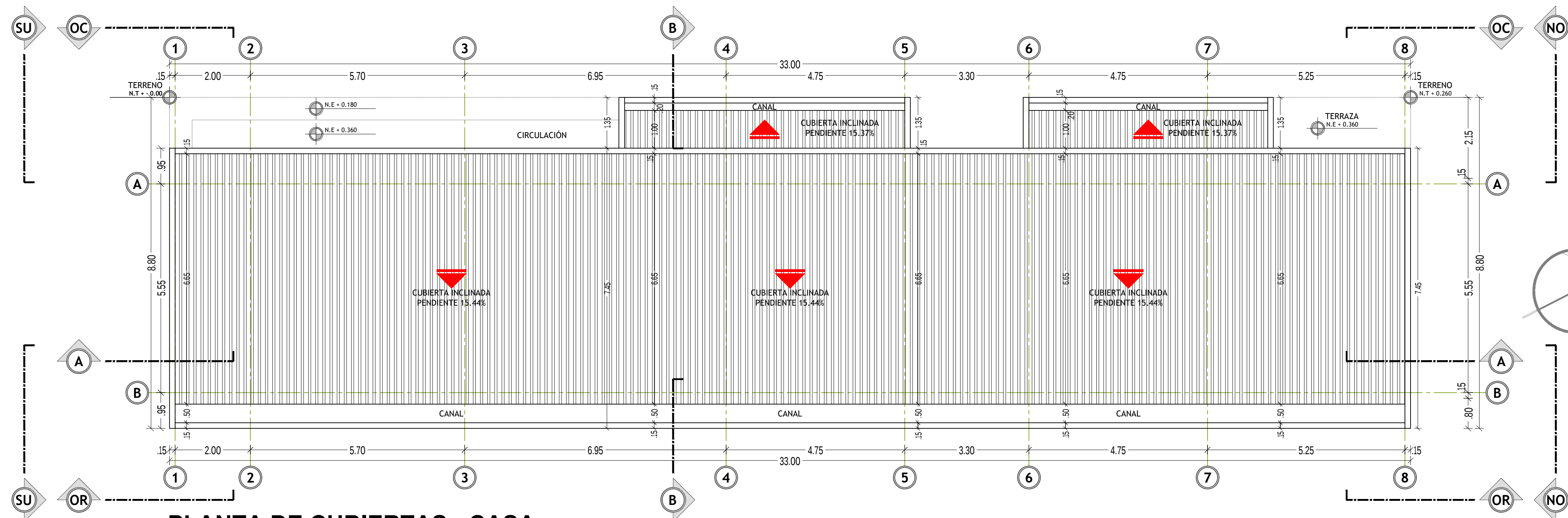
PLANTA DE CUBIERTAS - CASA
