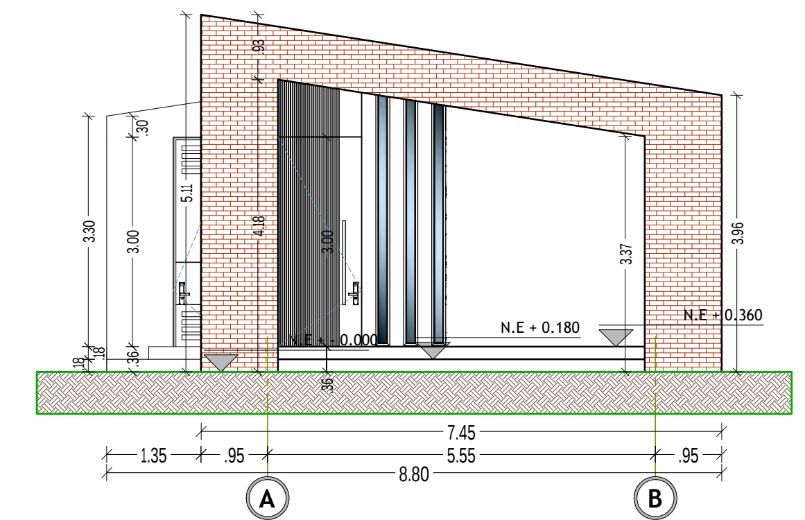
FACHADA SUROCCIDENTE - SU
