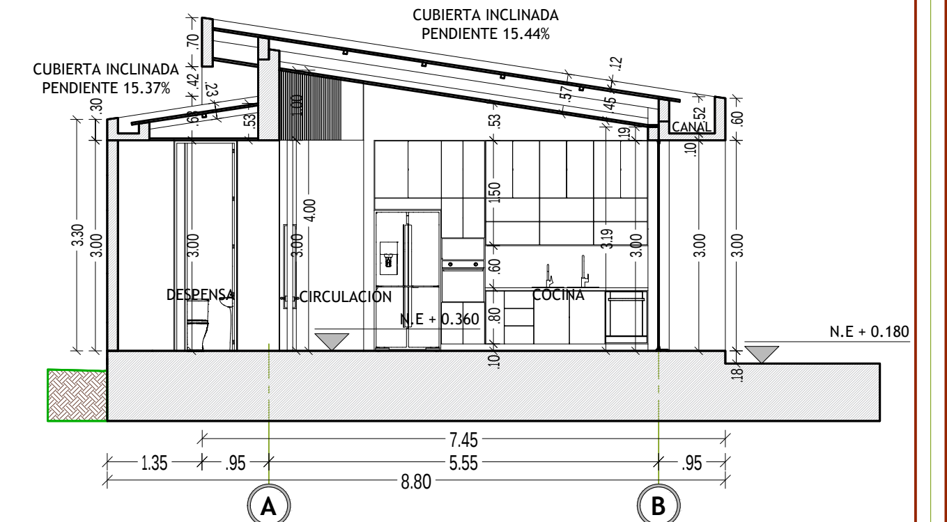
CORTE B-B
