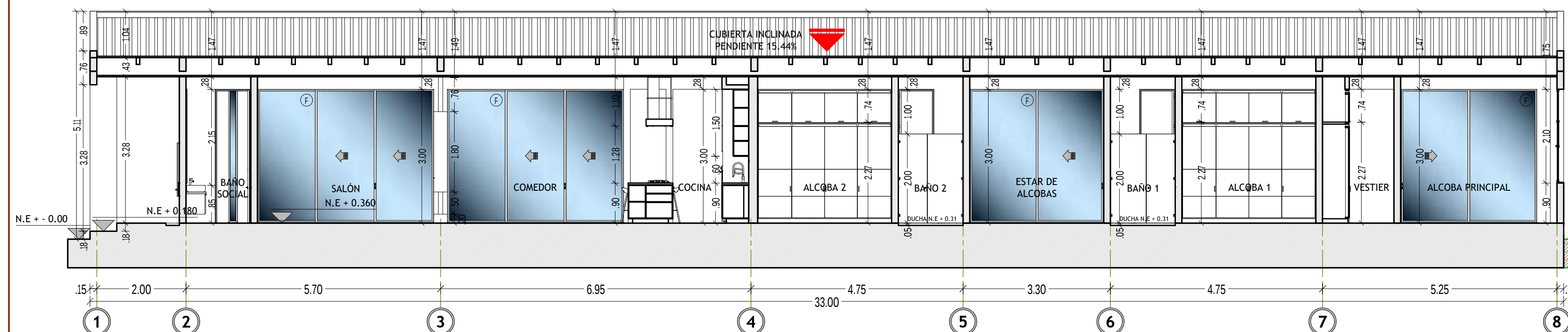
CORTE A-A
